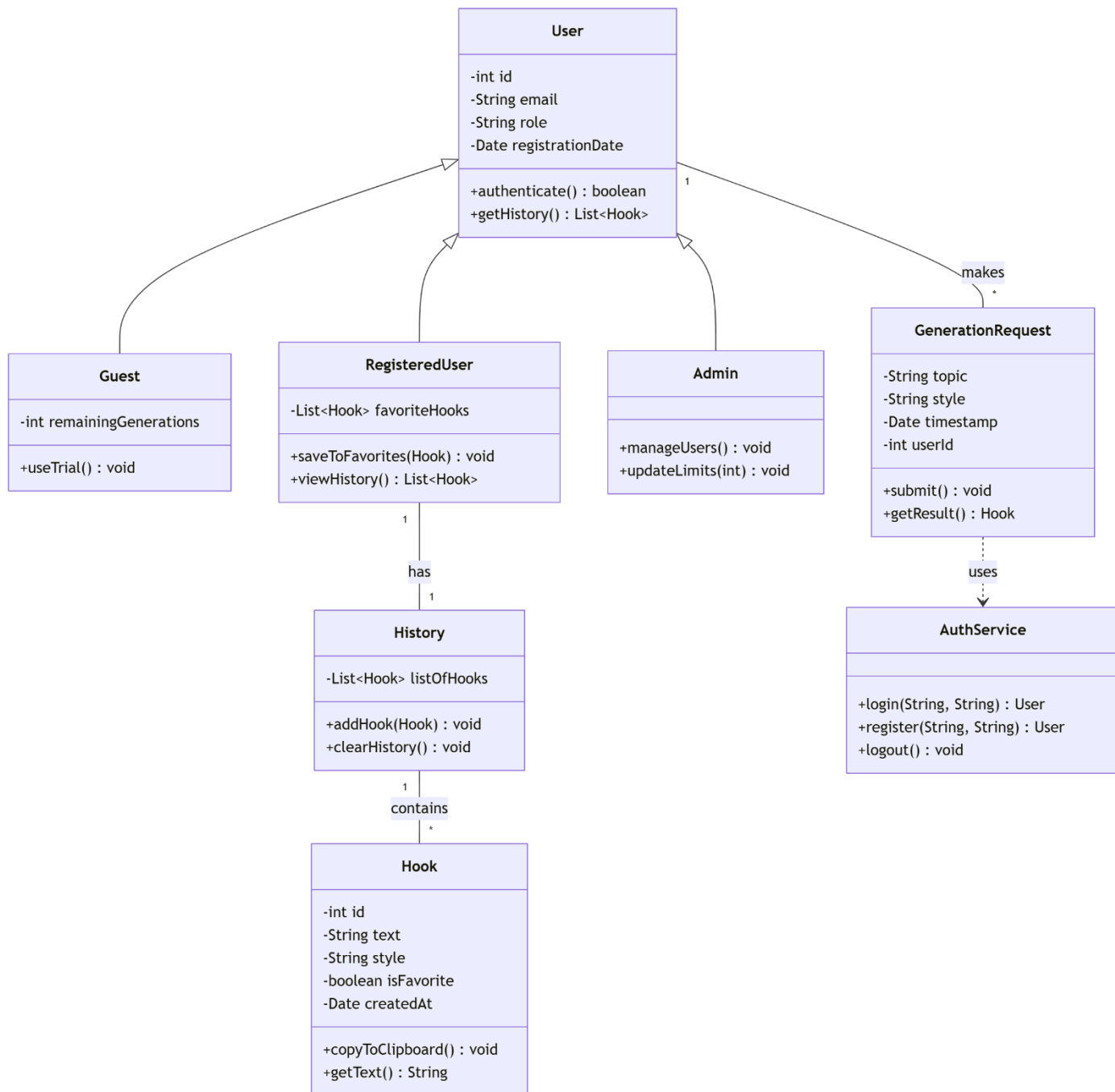
Рис. 2 – Діаграма класів.
