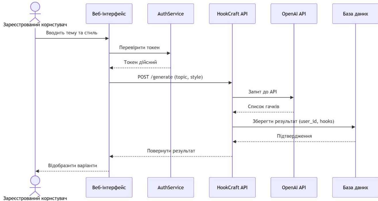
Рис. 3 – Діаграма послідовності.
