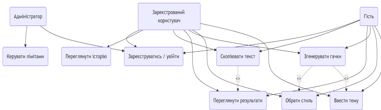
Рис. 1 – Діаграма прецедентів.
